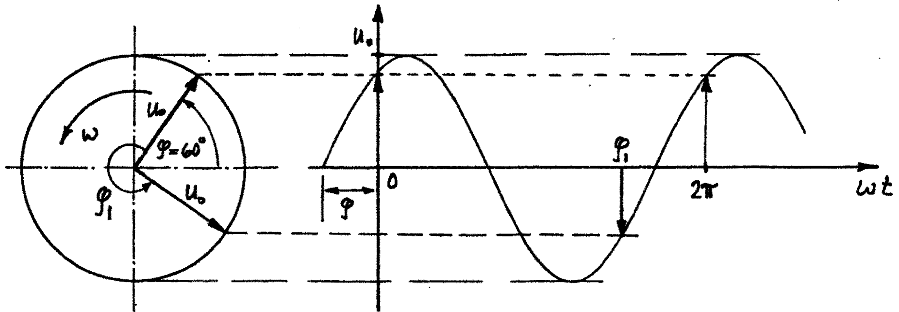
Zeigerdiagramm
